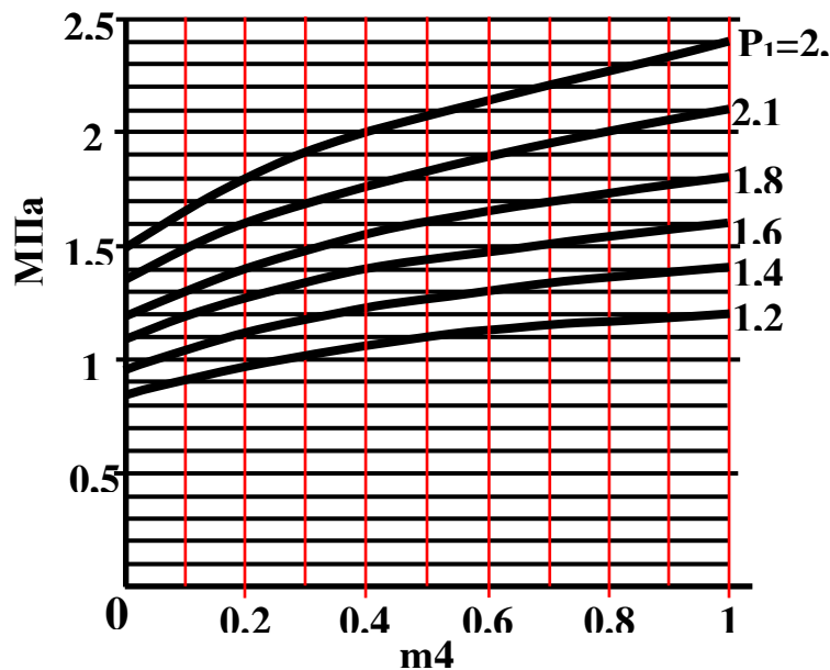
График для определения давления в изотермическом резервуаре в конце выпуска расчетного количества двуокиси углерода
