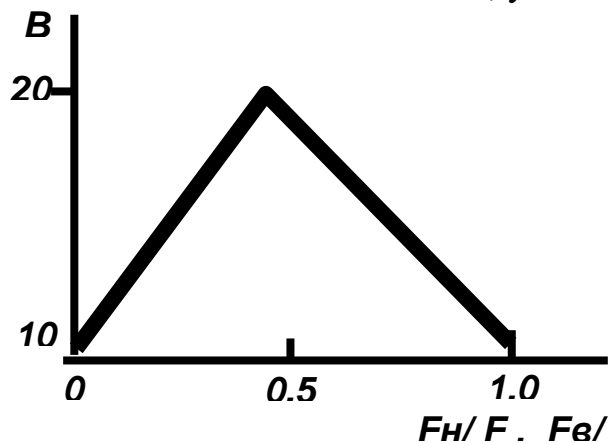
График для определения коэффициента B при расчете коэффициента k_4
