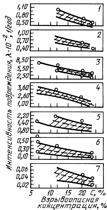
min и max \lambda - - - средние значения 1 — фланцы; 2 — задвижки; 3 — скрубберы; 4 — осушители; 5 — конденсаторы; 6 — емкости; 7 — трубы
